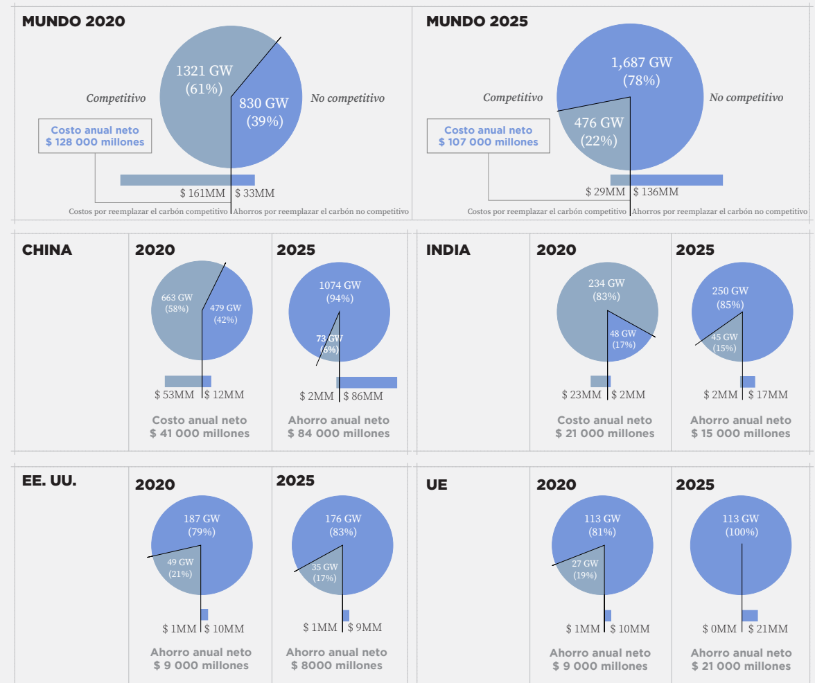
IMAGEN 2 Competitividad de los costos del carbón existente frente a las nuevas energías renovables y el almacenamiento
